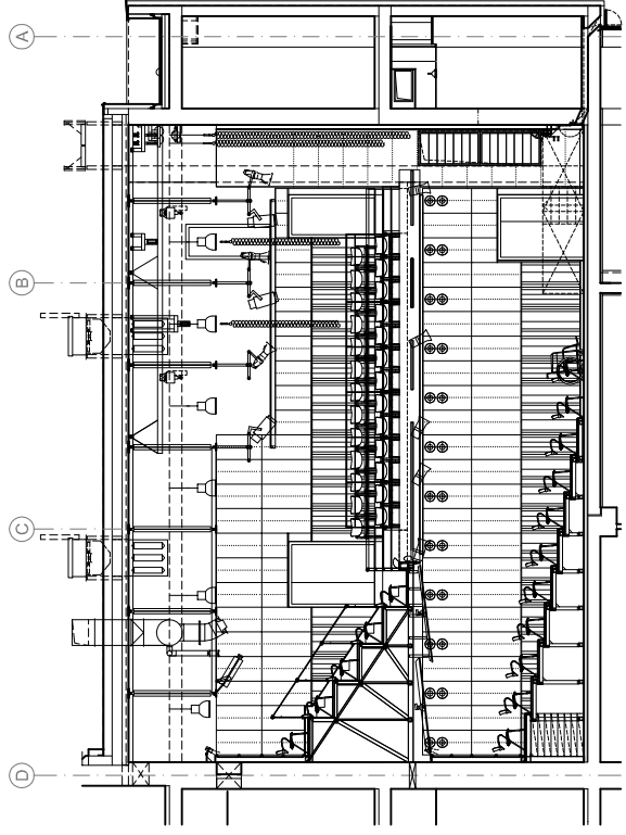
POZDĚLNÝ REZ
